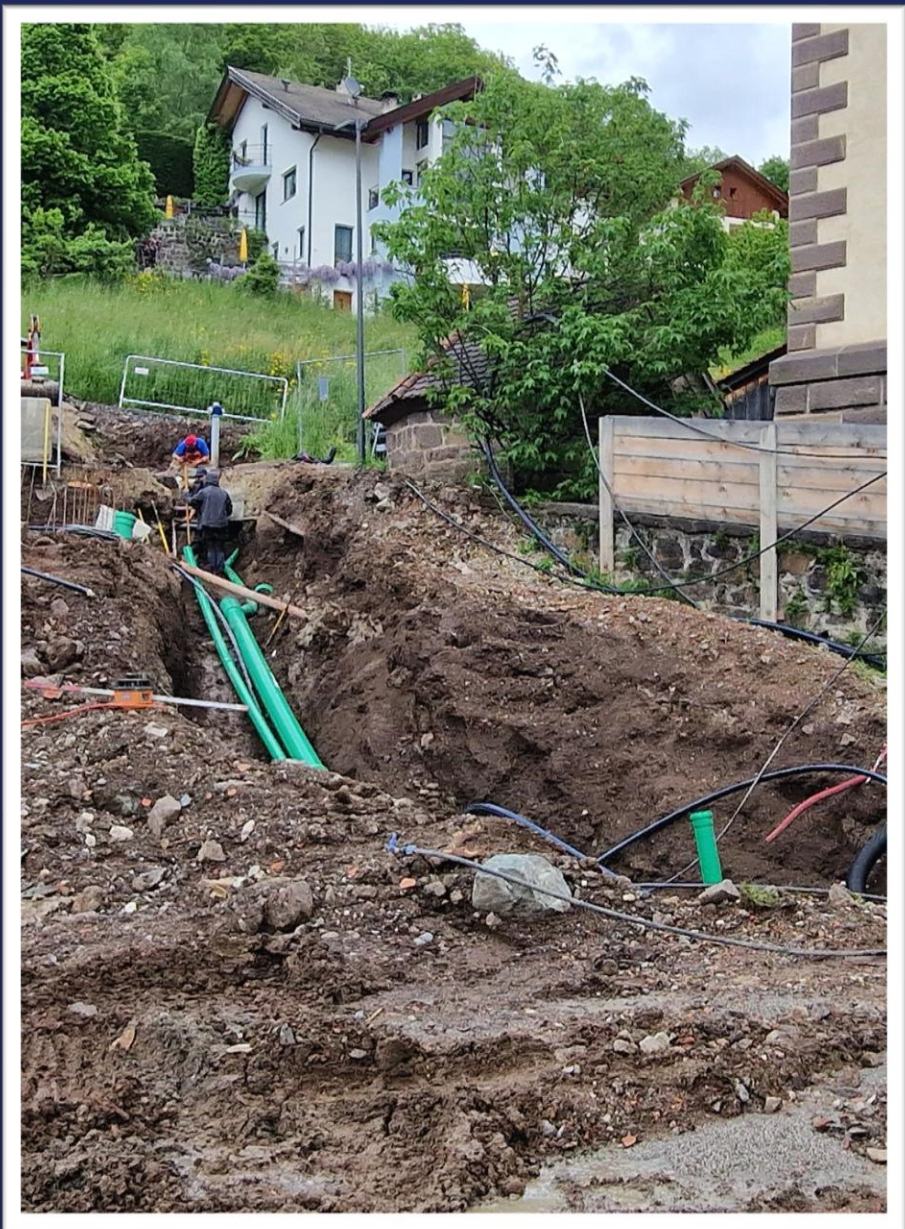
Neuverlegung der Infrastrukturen am Pfarrplatz Mitte Mai 2025
