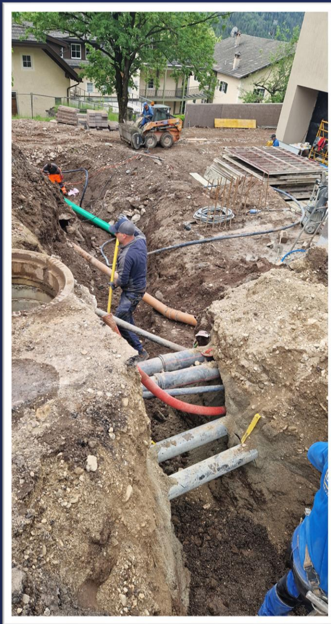
Neuverlegung der Infrastrukturen am Pfarrplatz Mitte Mai 2025
