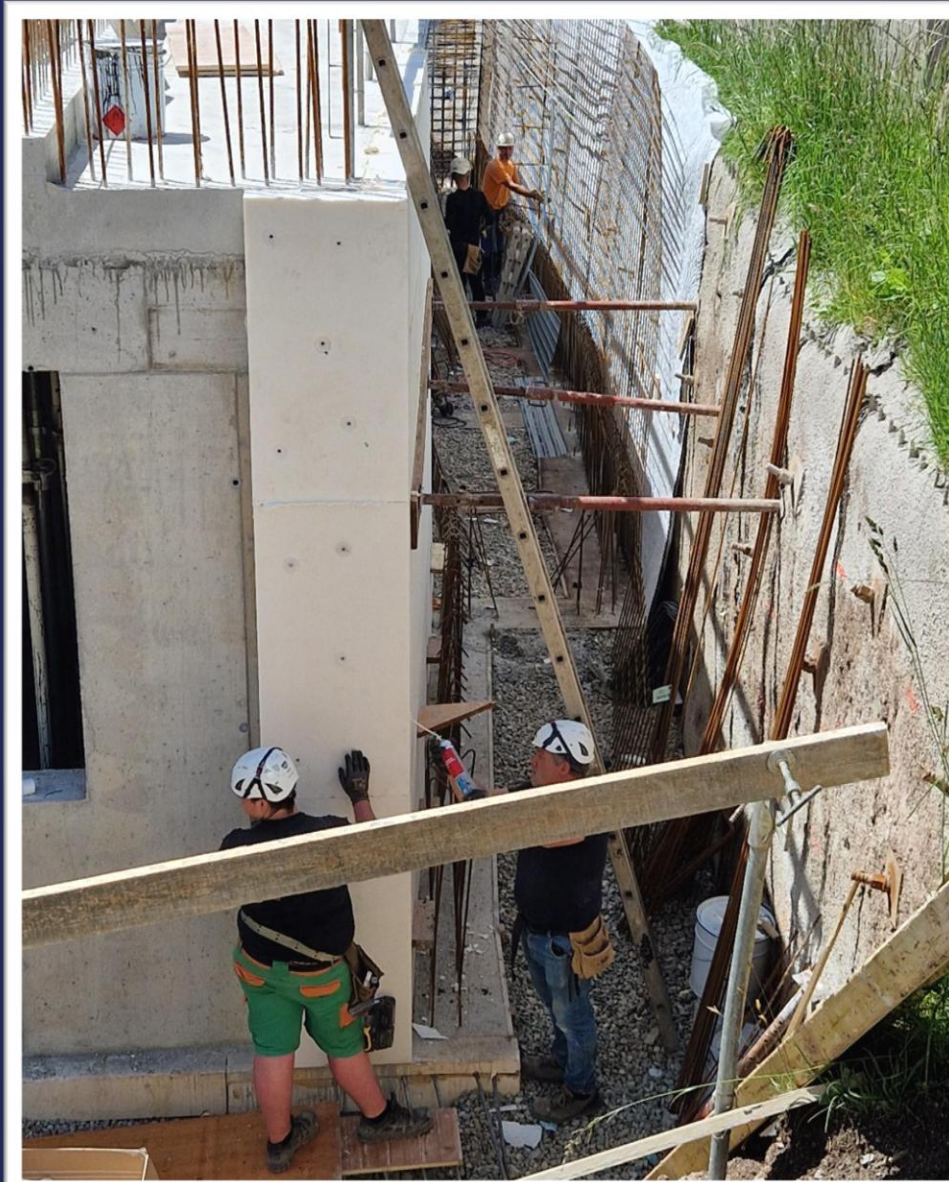
Vorbereitung der Stützmauer zur Straße am 29. Mai 2024
