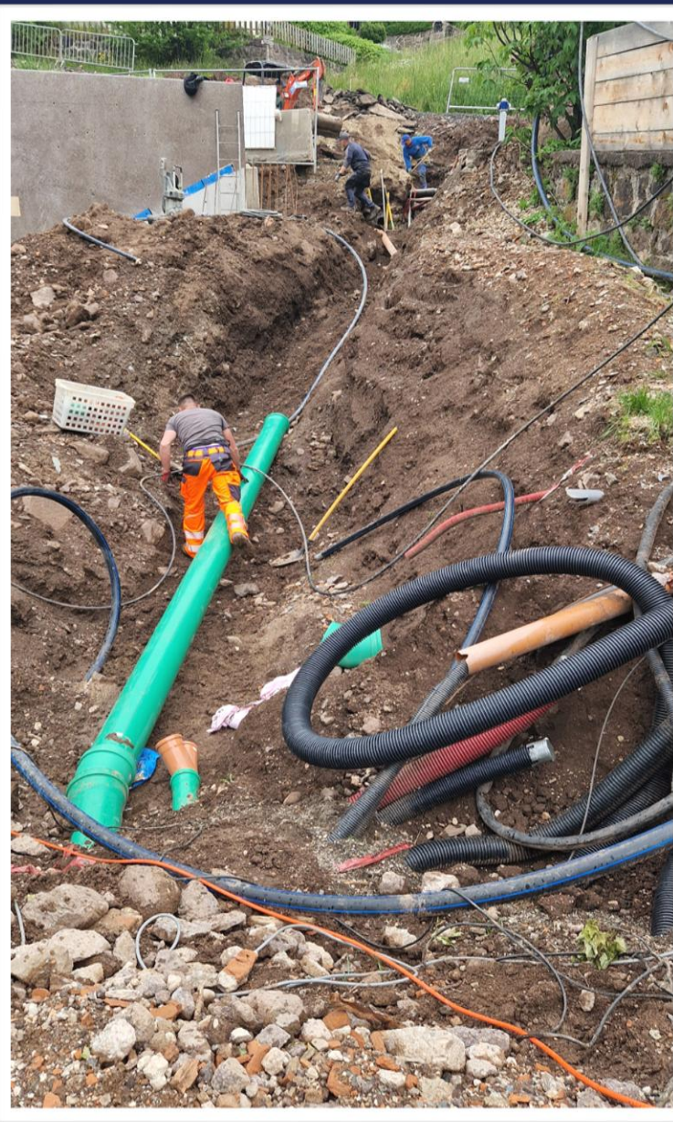
Neuverlegung der Infrastrukturen am Pfarrplatz Mitte Mai 2025
